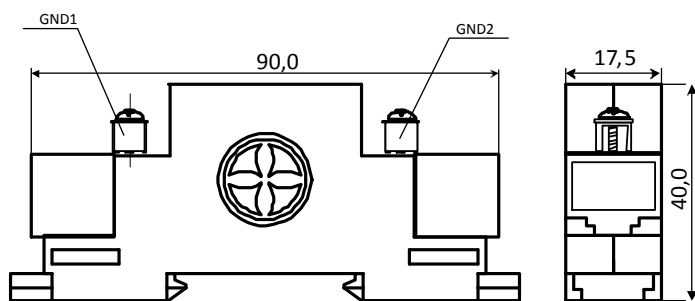
Рис.4 Габариты устройства
