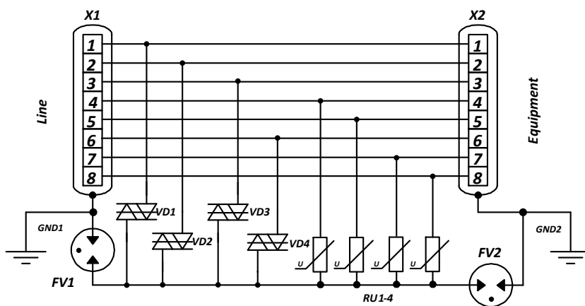
Рис.2 Схема принципиальная
